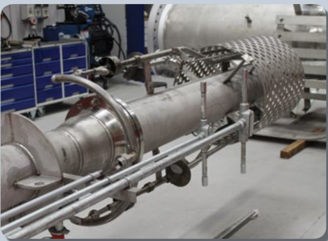
ZEECO Rental Flare
